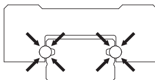
圖 2.3.3 哥德式 45^\circ 四方向負荷結構
