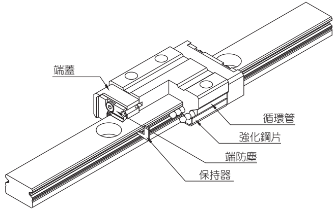
圖 2.3.4 TM 本體結構
