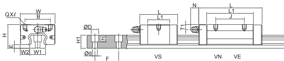
TRS-V 低組裝系列規格尺寸表
