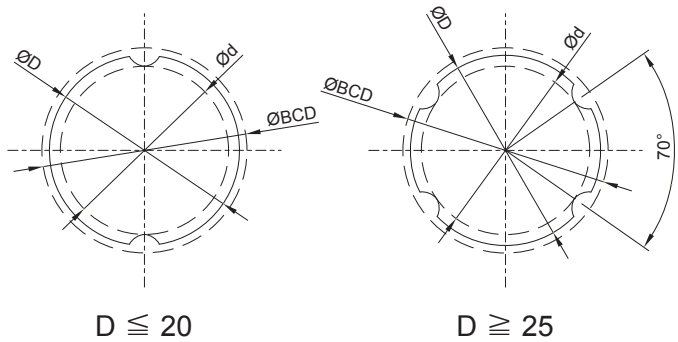
實心花鍵軸
