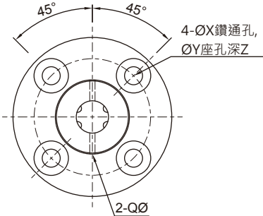
【四牙】型號：40、50
