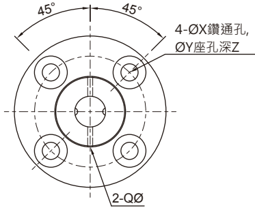
【二牙】型號：06、10、13
